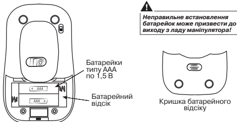
Мал. 4. Встановлення батарейок
